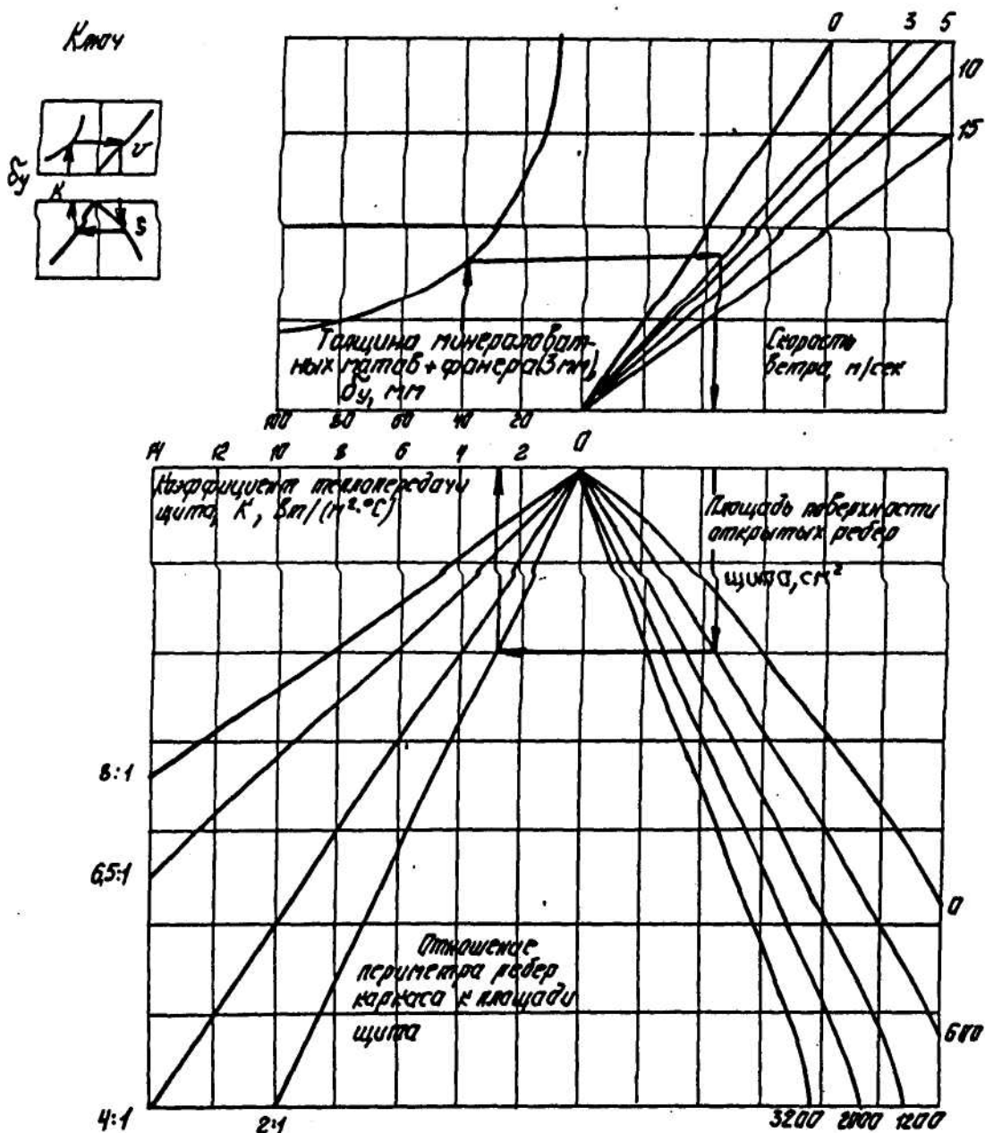
Рис.4. Номограмма для определения коэффициентов теплопередачи отелных опалубочных щитов
