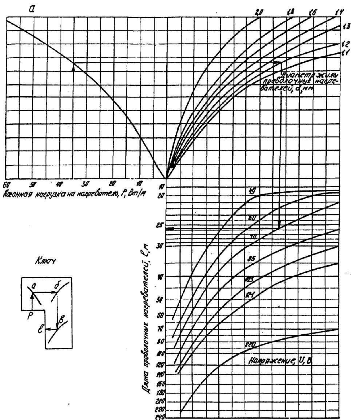
Рис. 8. Номограмма для определения длины проволочных нагревателей со стальной оцинкованной жилой
